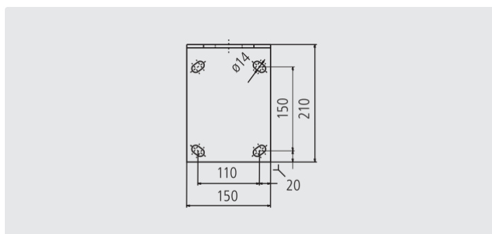
Płyta ścienna
