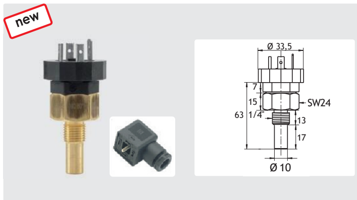
Bimetaliczny przełącznik temp. z wtyczką. Dokładność punktu przełączania ± 5° C. Reset temp. 15...40K. Napięcie przełączające do AC 250 V / 2A. Max. 10 bar na wlocie. Przełącznik 1/4" GZ
