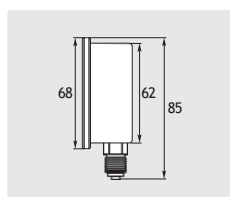
Ø 63 mm. 1/4" GZ. Obudowa stal nierdzewna. Wlot na dole. Typ WIKA
