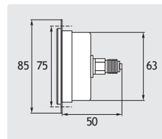
Ø 63 mm. 1/4" GZ. Z pierścieniem montaż. Obudowa stal nierdzewna. Wlot z tyłu
