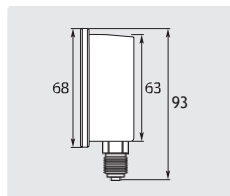
Ø 63 mm. 1/4" GZ. Obudowa stal nierdzewna. Wlot na dole
