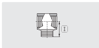
Mosiądz (T-block)
