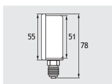
Ø 50 mm. 1/4" GZ. Obudowa stal nierdzewna. Wlot na dole
