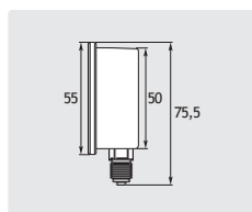
Ø 50 mm. 1/4" GZ. Obudowa stal nierdzewna. Wlot na dole. Typ WIKA
