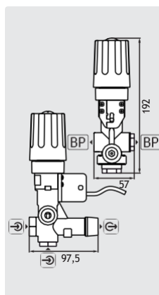
Trzpień reg
