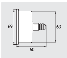
Ø 63 mm. 1/4" GZ. Obudowa stal nierdzewna. Wlot z tyłu
