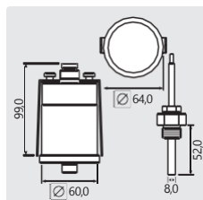
1/2" GZ. Styk 5 A - 250 V (ACI). Wskazanie temperatury 0 - 120 °C
