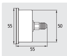
Ø 50 mm. 1/4" GZ. Obudowa stal nierdzewna. Wlot z tyłu. Typ WIKA
