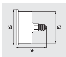
Ø 63 mm. 1/4" GZ. Obudowa stal nierdzewna. Wlot z tyłu. Typ WIKA
