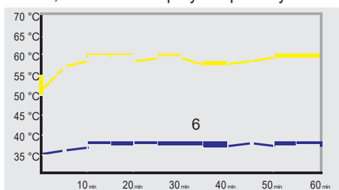
Temperatura powierzchni izolacji ST-28, ST-29 i ST-26 przy temp. wody 90 °C.
