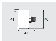
Ø 40 mm. 1/8" GZ. Obudowa plastik. Wlot z tyłu
