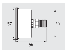
Ø 50 mm. 1/4" GZ. Obudowa stal nierdzewna. Wlot z tyłu
